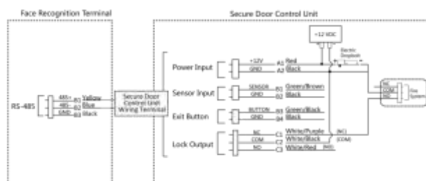
Рисунок 4-6 Подключение устройства
