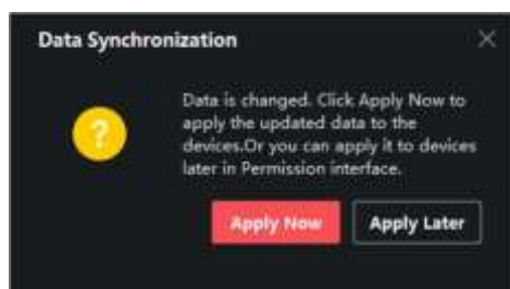
Рисунок 7-7 Синхронизация данных
