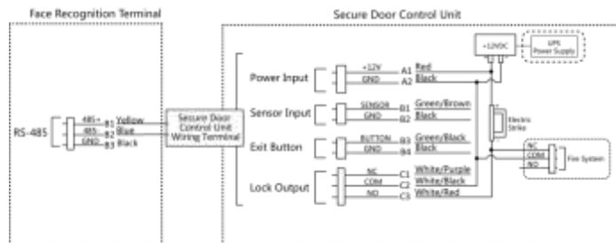
Рисунок 4- 8 Подключение устройства
