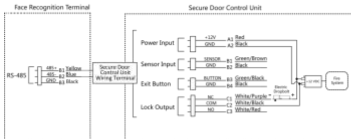
Рисунок 4-4 Подключение устройства
